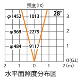
水平面照度分布図
