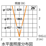
水平面照度分布図
