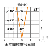
水平面照度分布図
