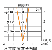
水平面照度分布図
