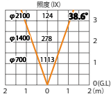
水平面照度分布図
